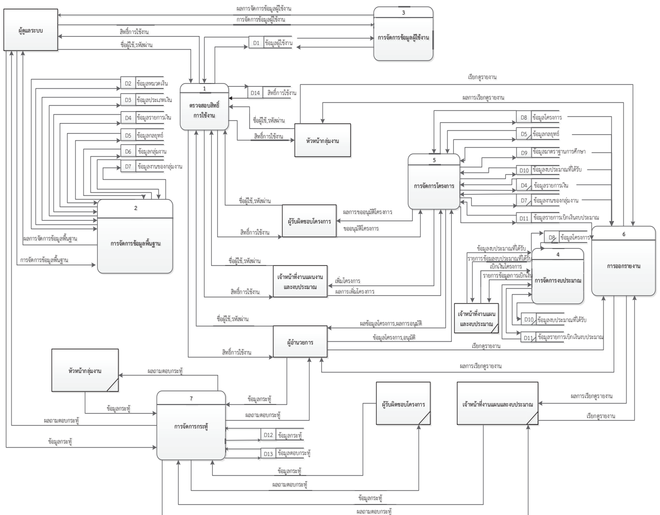
ภาพที่ 1 แผนภาพกระแสข้อมูลระดับ 0
